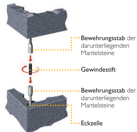
Bild 3 - Verschraubung
