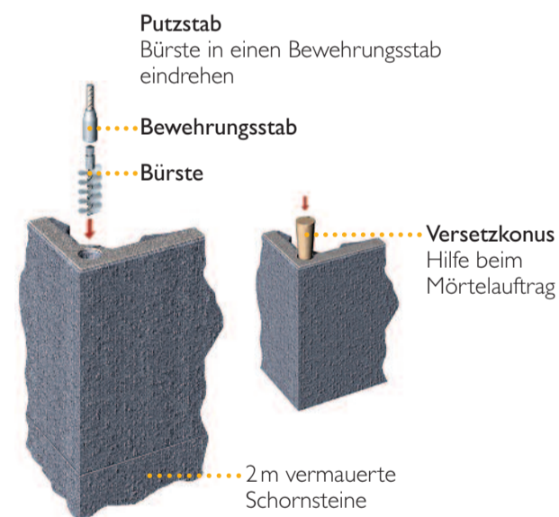
Bild 2 - Eckkanalreinigung
