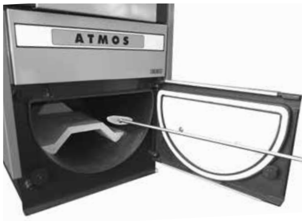
Geöffneter Unterraum des Kessels mit Dach und mit Vorführung der Ascheentleerung mittels Schürhakens
